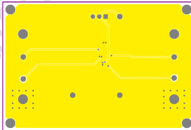
Figure 23. EVM BOTTOM Layer
