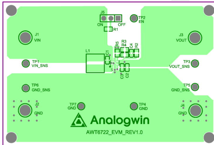
Figure 22. EVM TOP Layer
